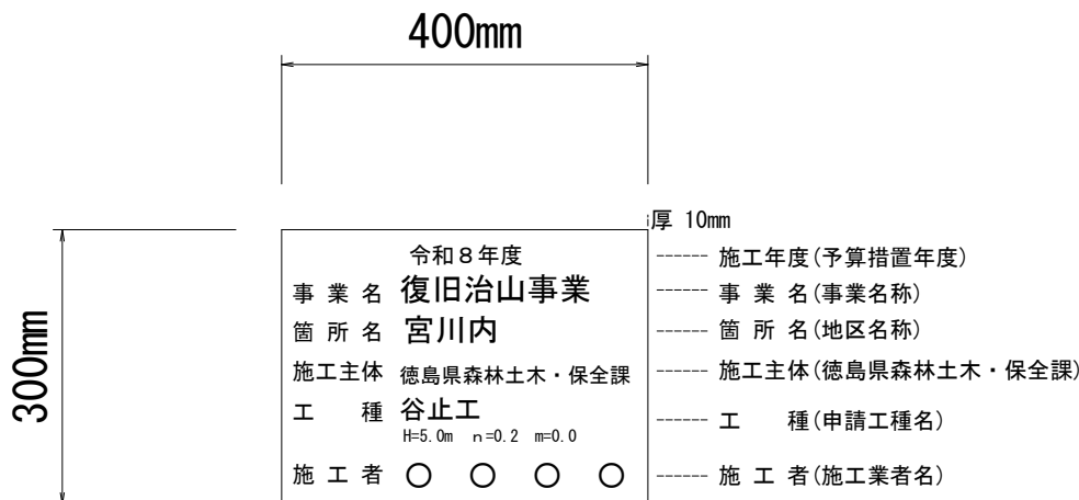
図1 銘板の寸法及び記載事項
